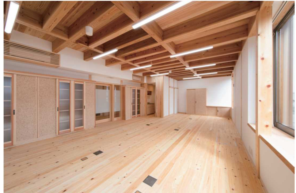
▲4m材プレカット加工 市販品の梁受け金物使用
